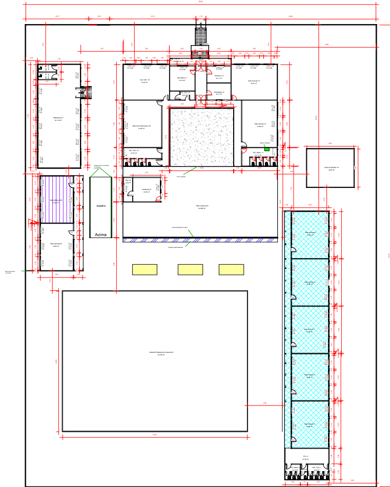
1 Planta Baixa 1 : 200
