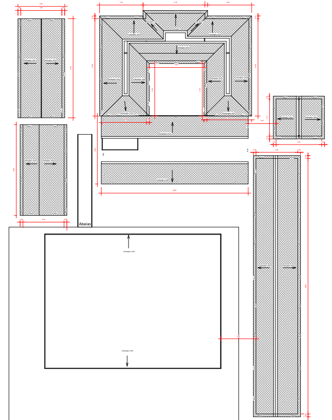
2 Tehado 1 : 200
